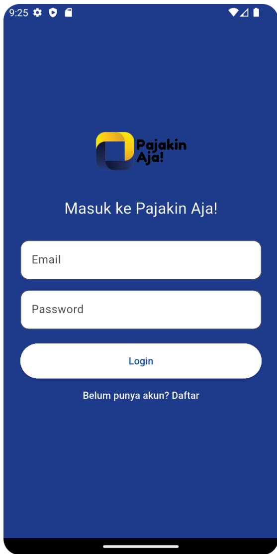
Gambar 3. Halaman login
